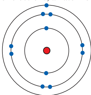
A sodium atom Fig. 10.1
